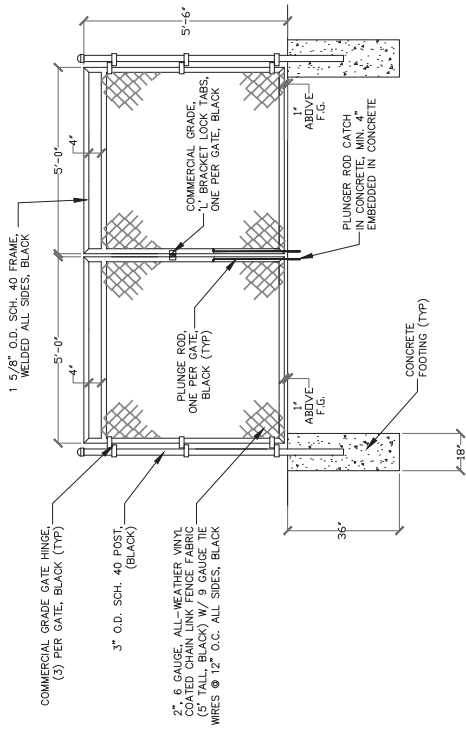
J 5'-6" MAINTENANCE GATE N.T.S
